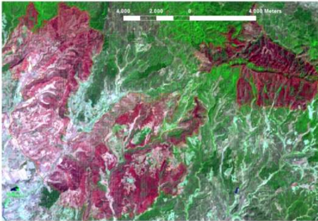
Imagen 1: Identificación de la superficie quemada en el año 1994 según imagen Landsat 5 TM, (RGB: 7;4;1)
