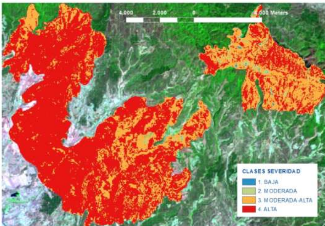
Imagen 2: Cartografía de severidad post-incendio según la inversión de modelos PROSPECT y GeoSail (DeSantis y Chuvieco, 2009).
